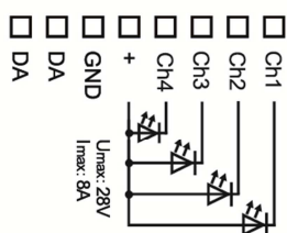
Anschlussplan 8A
