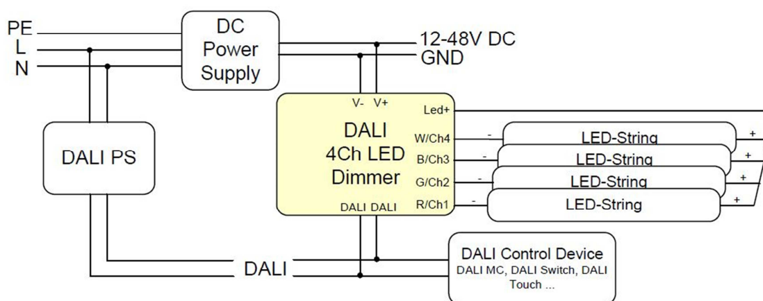
Prinzipschaltbild
