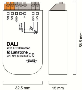
Geometrie 8A
