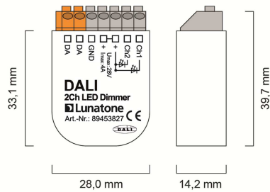
Geometrie 4A
