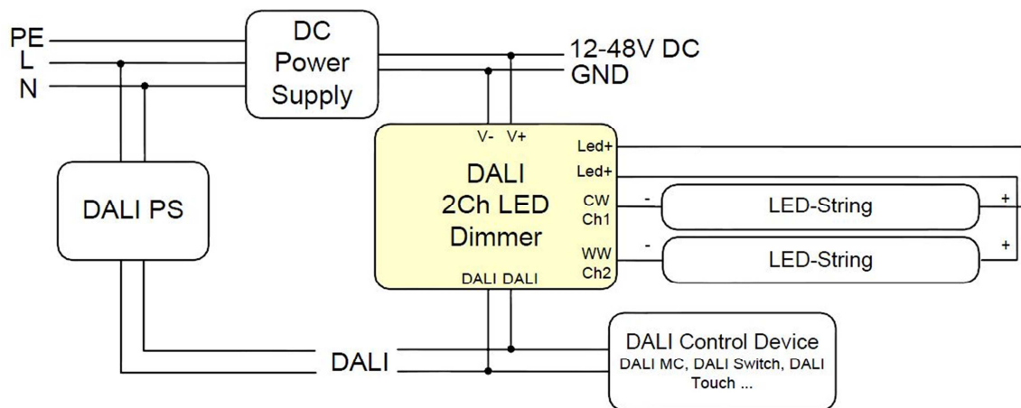
Prinzipschaltbild
